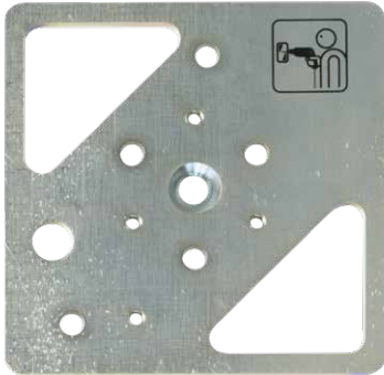
El principio de funciona- miento del sistema de alarma es la placa base para detectores de ruido inducido (KSM). Estos detectan los intentos de corte o taladra- do y dispara la alarma.
